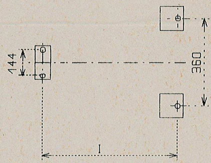
Anschlußstutzen DIN 2633 Connections
